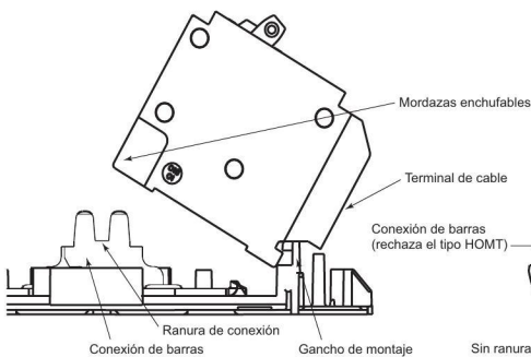
Figura 1: Interruptor automático HOM o HOMT
